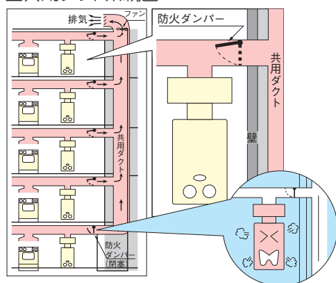
■共用ダクト系統図
